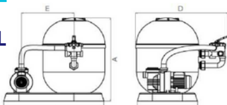
Dimensiones GFT
